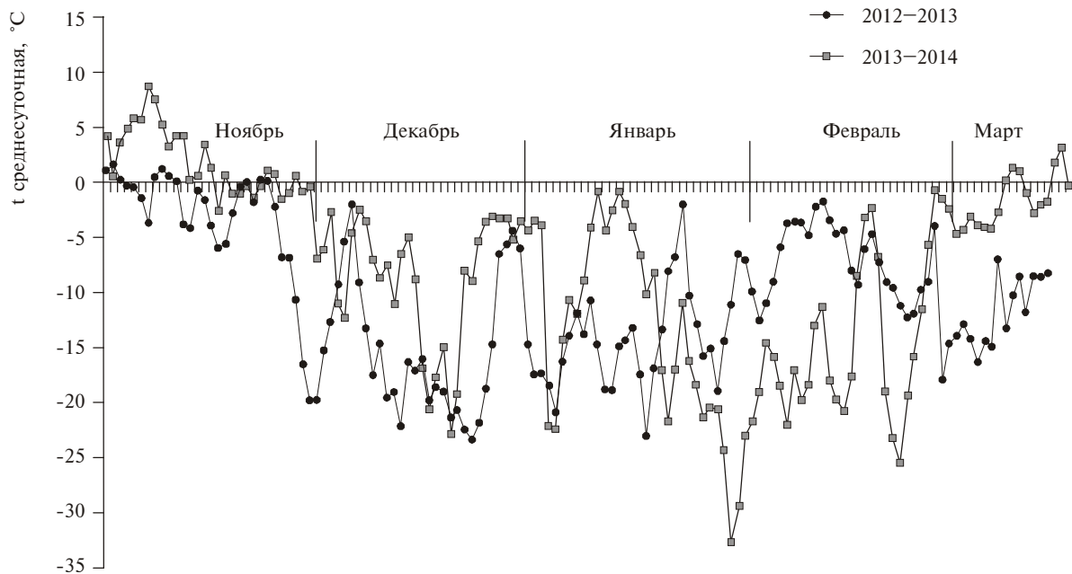
Рис. 1. Динамика среднесуточных температур в течение холодных периодов 2012–2013 и 2013–2014 гг. по данным метеостанции г. Сысерть (Свердловская обл.).
