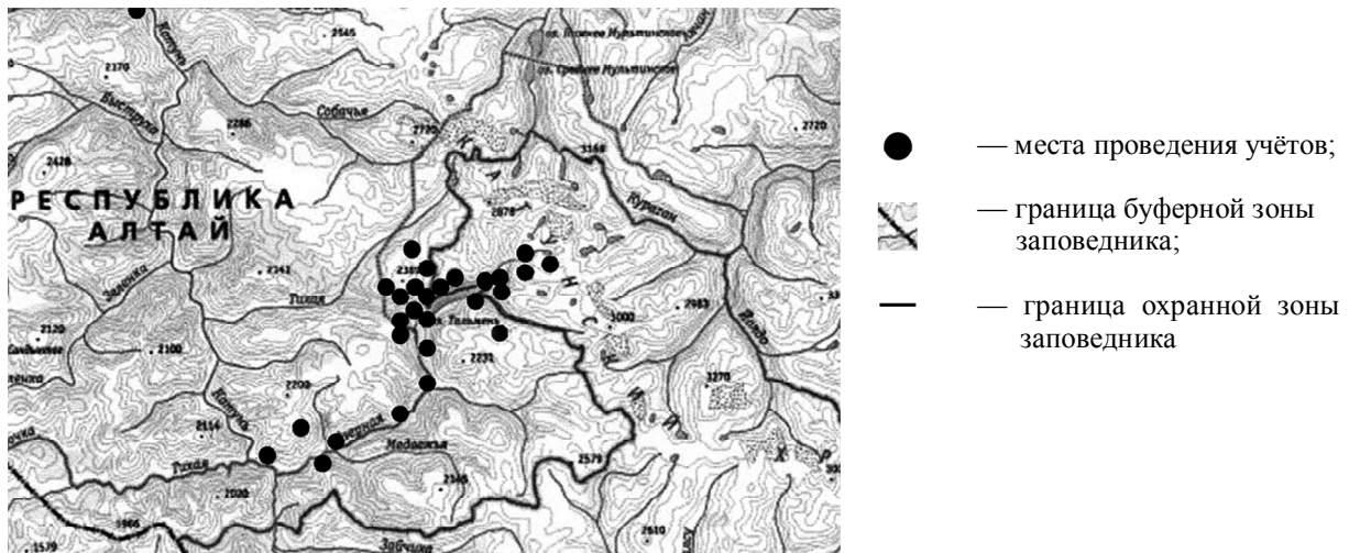
Рис. 1. Пункты сбора материала по цикадовым на территории ГПЗ «Катунский» и его окрестностей.
