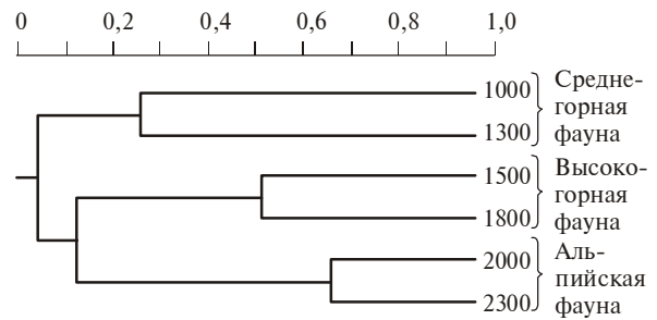
Рис. 2. Кластерная диаграмма сходства населения цикадовых различных поясов. По горизонтали — индекс Чекановского-Сёренсена, рассчитанный по количественным данным, по вертикали — абсолютная высота (м н.у.м.).
