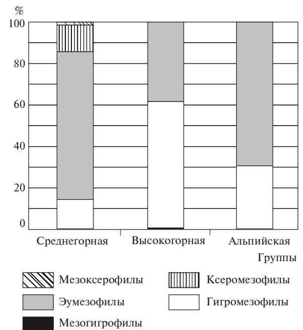
Рис. 3. Распределение гигрогрупп цикадовых в зависимости от высоты (м н.у.м.).
